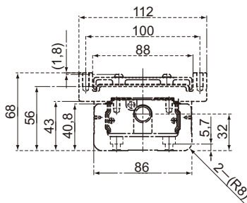
Поперечный разрез В-В
